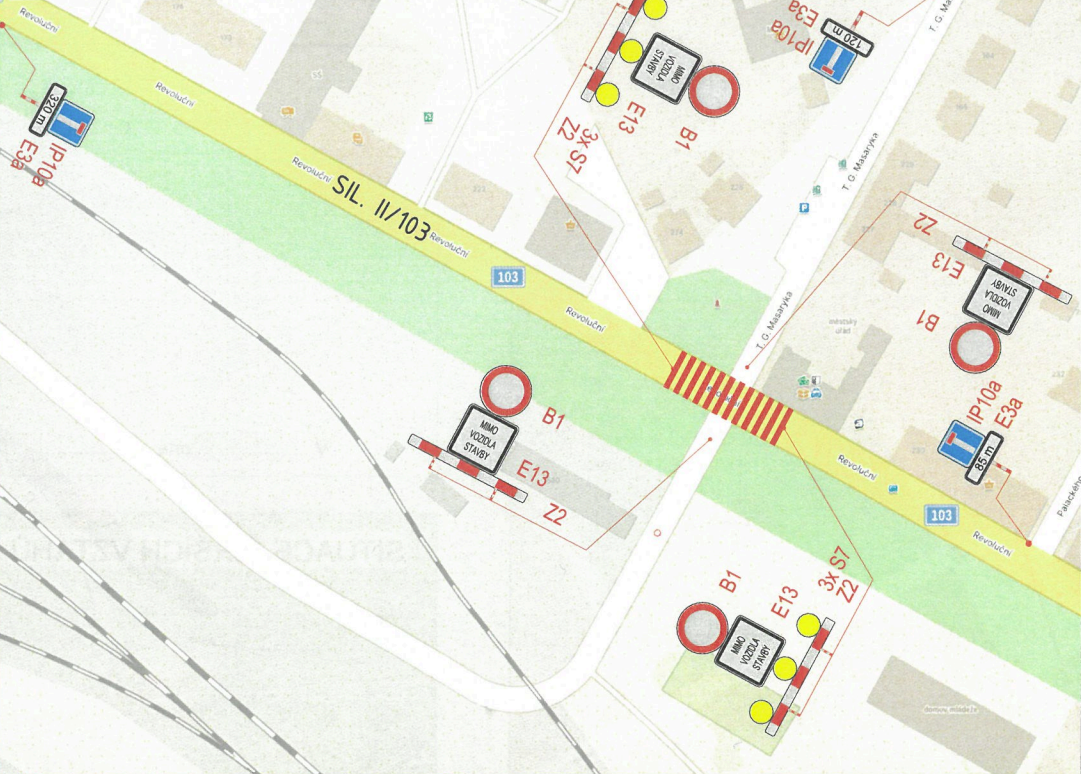
SITUACE DIO - DETAIL
